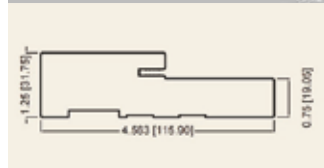
4-9/16" JAMB
